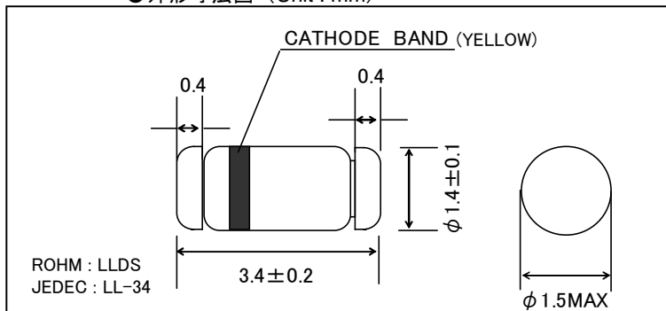
●ランド寸法図 (Unit : mm)
